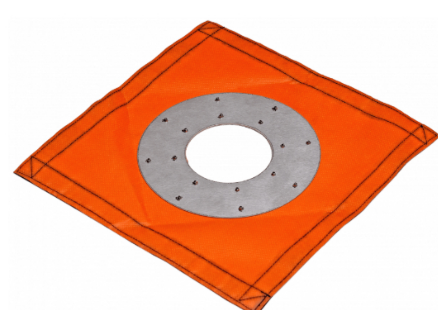
Вырез под трубу
